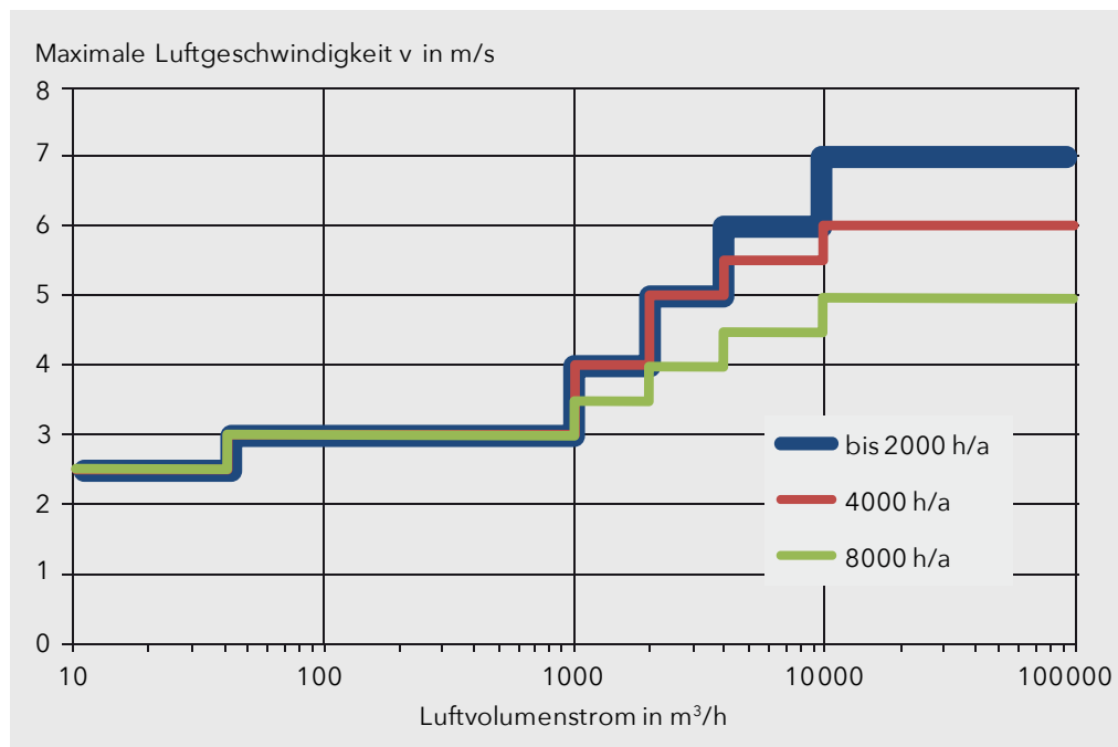
Abbildung 7: Maximale Luftgeschwindigkeiten in runden Luftleitungen
