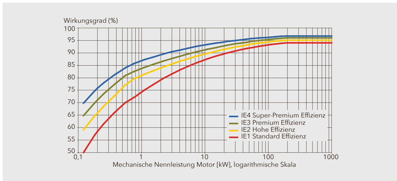
Abbildung 3: Wirkungsgrade von Elektromotoren (4 Pole, 50 Hz), gemäss IEC 60034-30-1
