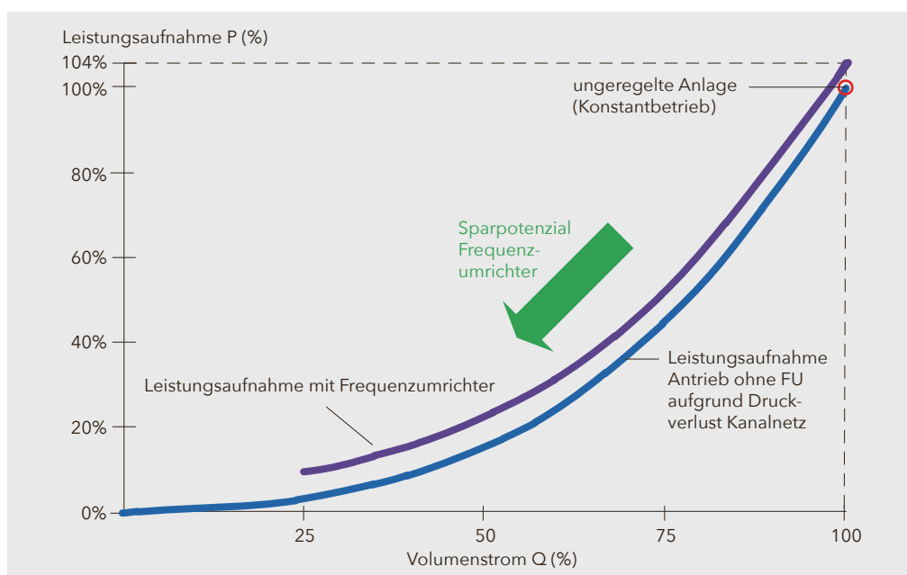
Abbildung 5: Einsparpotential bei Ventilatoren mit Frequenzumrichtern (FU) respektive elektronisch kommutierten Motoren.
