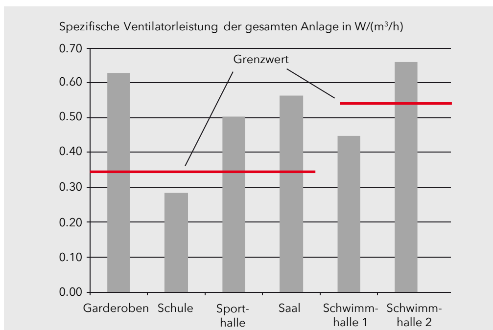
Abbildung 12: Beispiele von gemessenen spezifischen Ventilatorleistungen
