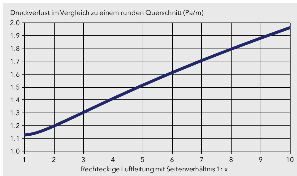
Abbildung 8: Druckverlust einer rechteckigen Luftleitung je nach Seitenverhältnis im Vergleich zu einer runden Luftleitung bei gleicher Luftgeschwindigkeit
