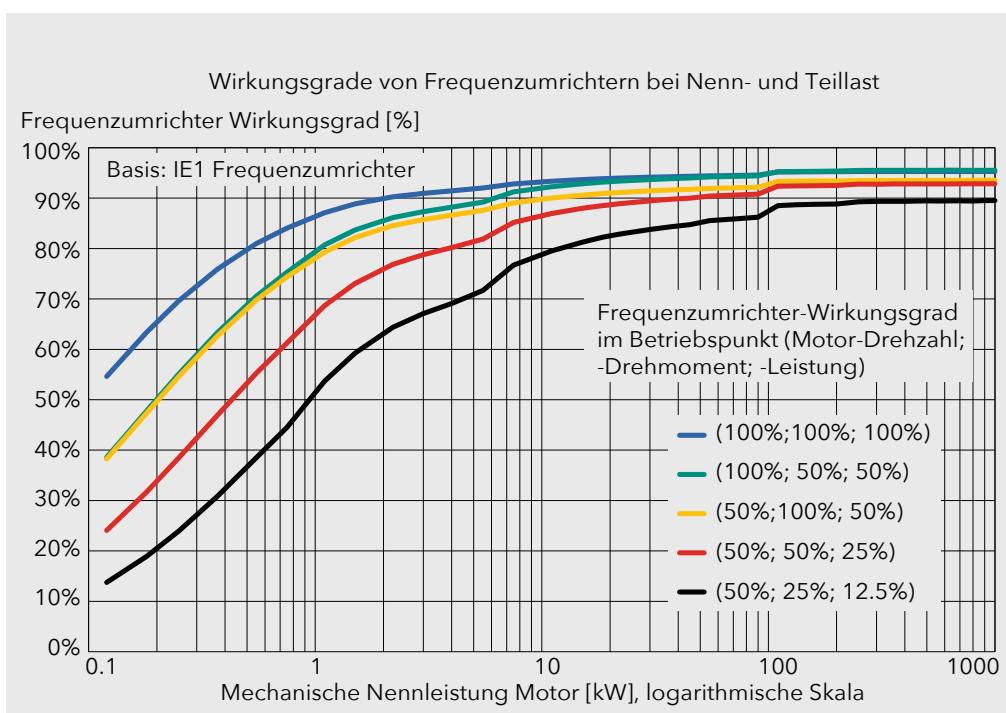
Abbildung 6: Wirkungsgrade von Frequenzumrichtern im Vergleich bei Nenn- und Teillast in Abhängigkeit der Motor-Nennleistung, nach IEC 61800-9-2, Edition 1, Basis: Effizienzklasse IE1 für Frequenzumrichter. Die Abbildung zeigt, dass ein FU bei tiefer Drehzahl beziehungsweise tiefem Drehmoment einen deutlichen Abfall des Wirkungsgrades, gegenüber des Wirkungsgrades bei Nennleistung, erleidet.
